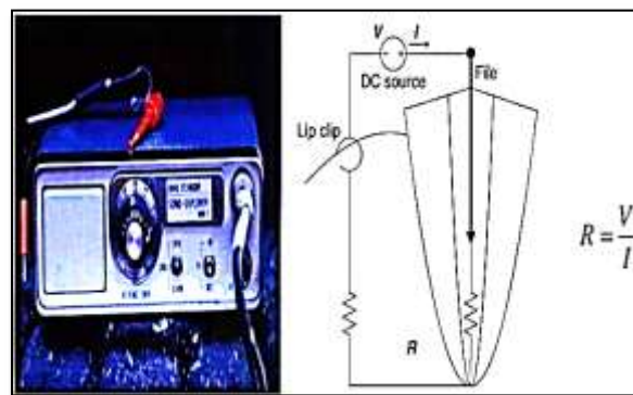
Fig. 2: Root Canal Meter
